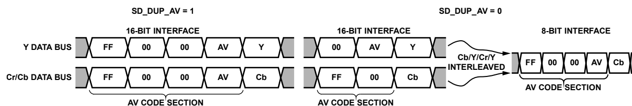
Figure 31. AV Code Duplication Control (64-Lead LQFP Only)
